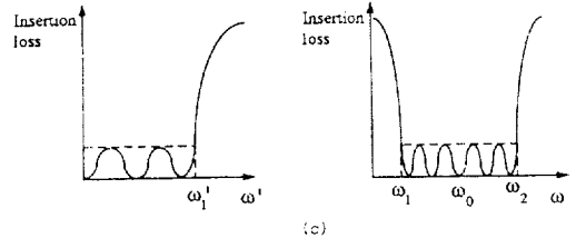
그림 4. 저역,대역 통과 필터의 기본 회로 및 감쇠 특성.
