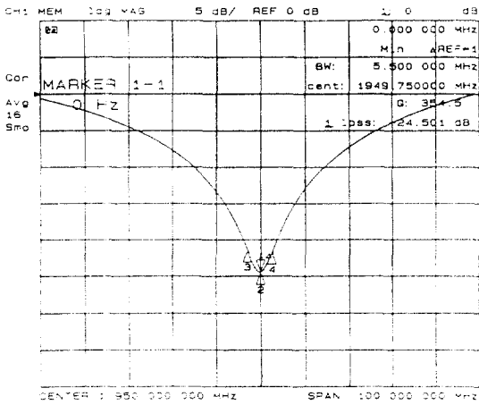
그림 9. \lambda/4 TEM 모드 유전체 공진기의 부부하 - Q.
