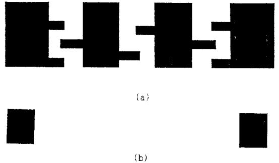
그림 8. 수신 필터의 캐패시턴스 구조 (a) 전 면 (b) 후 면 Fig. 8. Capacitance structure of receiving filter (a) Front side (b) Back side
