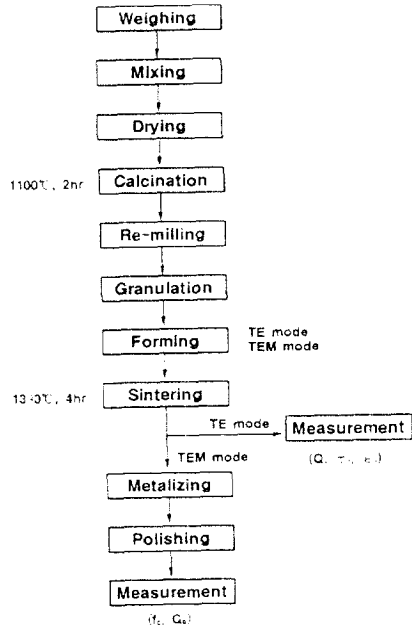
그림 2. \lambda/4 TEM 모드 유전체 공진기의 제조 공 정도.
