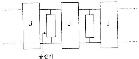
그림 5. J-인버터를 포함한 대역 통과 필터의 기본 회로.
