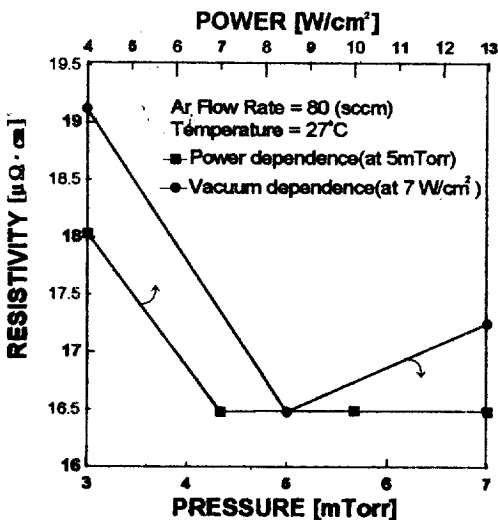
그림 2. 입력 power 및 Ar 가스압력 증가에 따른 Pt 박막의 비저항 변화.
