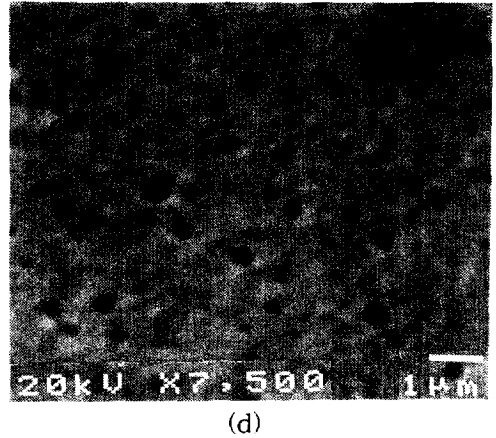
그림 6. 1000 °C에서 열처리를 (a) 거치지 않은 시료, (b) 60분, (c) 120분, (d) 240분 기간 Pt 박막의 SEM 표면 사진.
