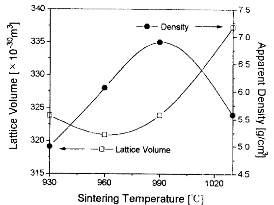
그림 3. 소결온도에 따른 BiNbO 4 시편의 격자 체적 및 소결밀도
