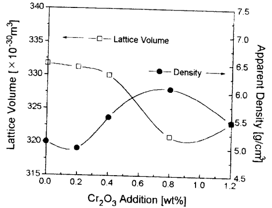
그림 2. Cr 2 O 3 첨가량에 따른 BiNbO 4 시편의 격자 체적 및 소결밀도
