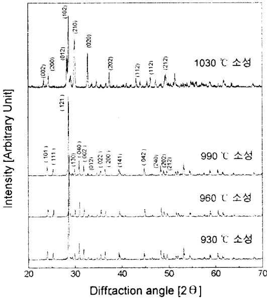
그림 1. 소결온도에 따른 BiNbO 4 시편의 X-RD peaks
