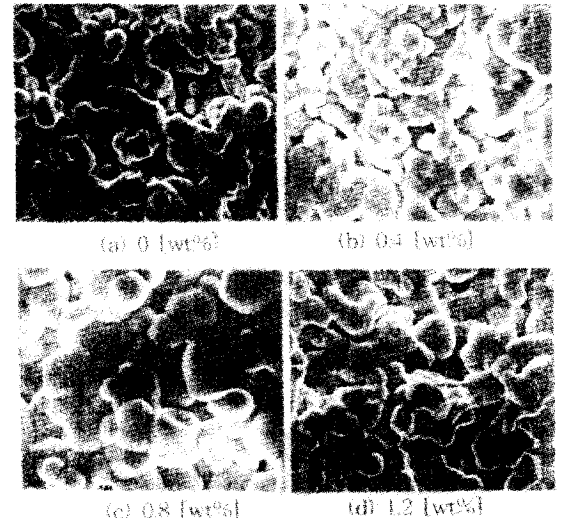
사진 2. 소성온도에 따른 BiNbO_4 시편의 미세구조 ( 0.8 [wt%] Cr_2O_3 첨가 )
