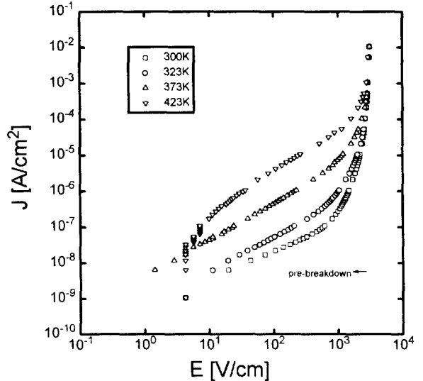
그림 9. 여러 가지 온도에서의 J-E 특성 곡선(B 조성)
