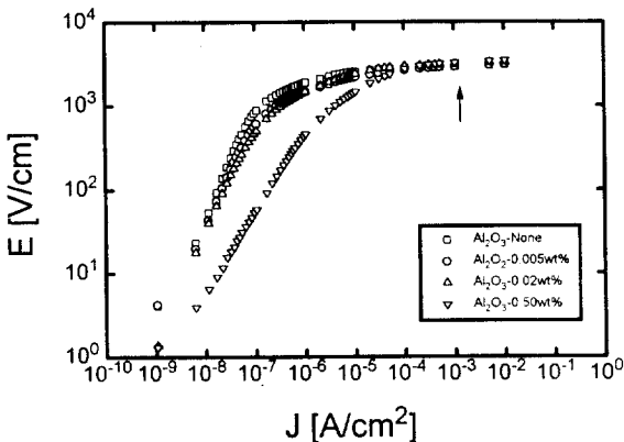
그림 6. ZnO 바리스터의 J-E 특성곡선 Fig. 6. Plot of J-E characteristics of ZnO samples
