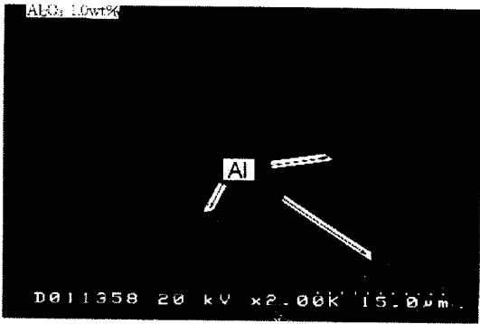
그림 5. 스피넬상(ZnAl 2 O 4 )에 편석된 Al-K \alpha X-ray 이미지(Al 2 O 3 1.0wt%) Fig. 5. Al-K \alpha X-ray image in the spinel phase(ZnAl 2 O 4 ) (Al 2 O 3 1.0wt%)
