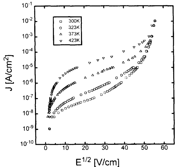
그림 10. 항복 전영역에서의 J-E 1/2 특성의 온도 의존성(B조성)
