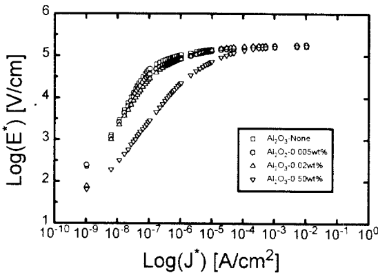
그림 7. 입자크기에 따라 정규화된 J-E 특성곡선 Fig. 7. Normalized J-E characteristics of ZnO samples with the grain size
