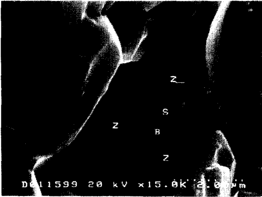
그림 3. SEM 조직사진 (B조성, Z:ZnO입자 B:Bi 입자 S:스피넬상)
