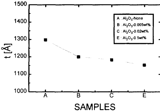
그림 8. Al 2 O 3 첨가량에 따른 공핍층 두께 변화 Fig. 8. The thickness of depletion layer with Al 2 O 3 additions
