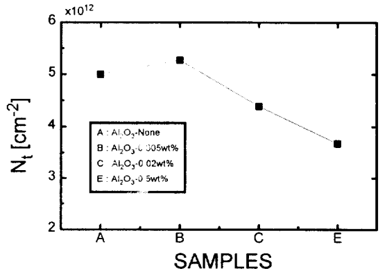
그림 14. Al 2 O 3 첨가량에 따른 계면결함밀도 N i 의 변화
