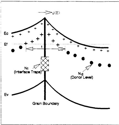
그림 1. 입계에 형성된 이중전위장벽의 에너지 준위 구조 Fig. 1. Energy level of double Schottky barrier at the grain boundary
