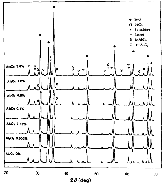
그림 4. 제조 시편의 XRD 곡선 Fig. 4. XRD curve of ZnO samples
