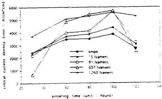
그림 4. 프레싱된 선재의 열처리 시간에 따른 임계 전류 밀도 (a) 단심 (b) 15 심 (c) 91 심 (d) 637심 (e) 1260 심
