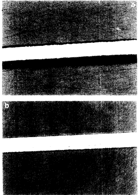
그림 3. 1260심 테이프의 절단 방향에 따른 내부 구조
