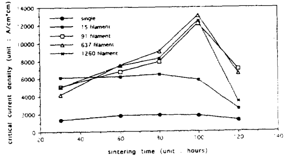
그림 5. 로울링된 선재의 열처리 시간에 따른 임계 전류 밀도 (a) 단심 (b) 15 심 (c) 91 심 (d) 637 심 (e) 1260 심
