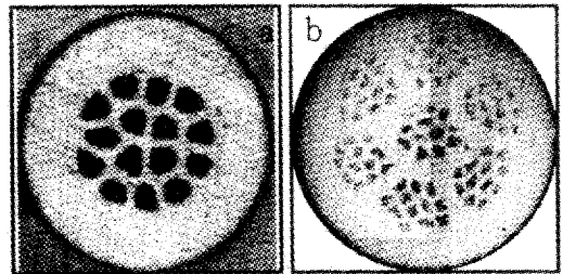
그림 1. 지름 1mm까지 성형된 고온 초전도 다심 선재의 단면 (a) 15 심 (b) 1260 심 Fig. 1. Cross section of 1mm diameter multi-layer superconductor wire. (a) 15 filaments (b) 1260 filaments
