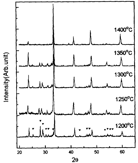
그림 1. 0.7CaTiO 3 -0.3LaAlO 3 의 하소 온도 변화에 따른 X-선 회절 모양
