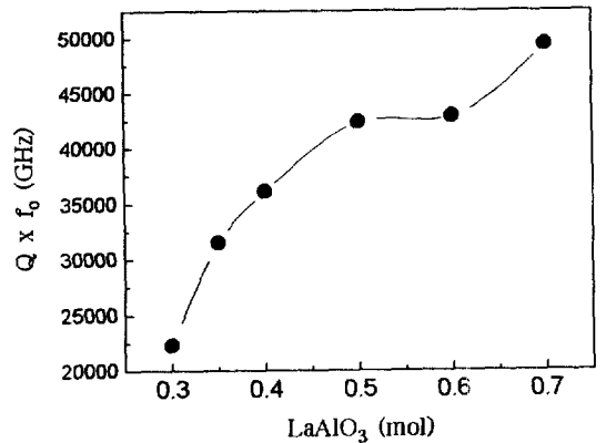
그림 8. 1600°C에서 4시간 소결된 (1-x)CaTiO 3 -xLaAlO 3 의 Q·f 0 .
