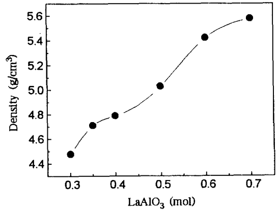
그림 5. 1600°C에서 4시간 소결된 (1-x)CaTiO 3 -xLaAlO 3 의 밀도 변화
