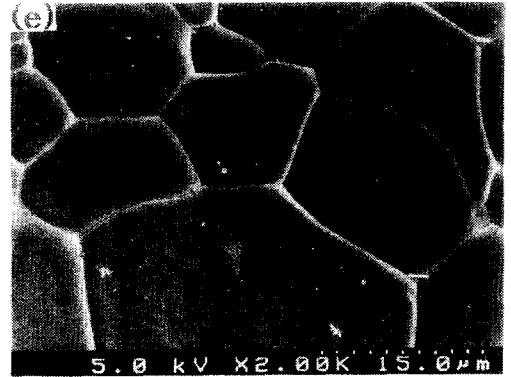
그림 4. 1600°C에서 4시간 소결된 (1-x)CaTiO 3 -xLaAlO 3 의 미세구조
