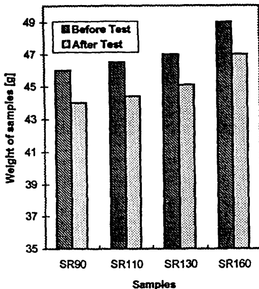
그림 8. 시료들의 무게 손실 Fig. 8. Weight loss for samples
