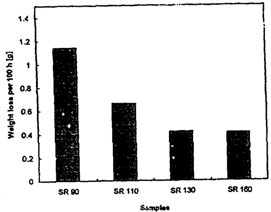
그림 9. 100 시간 당 시료의 무게 손실 Fig. 9. Weight loss per 100 h for specimen
