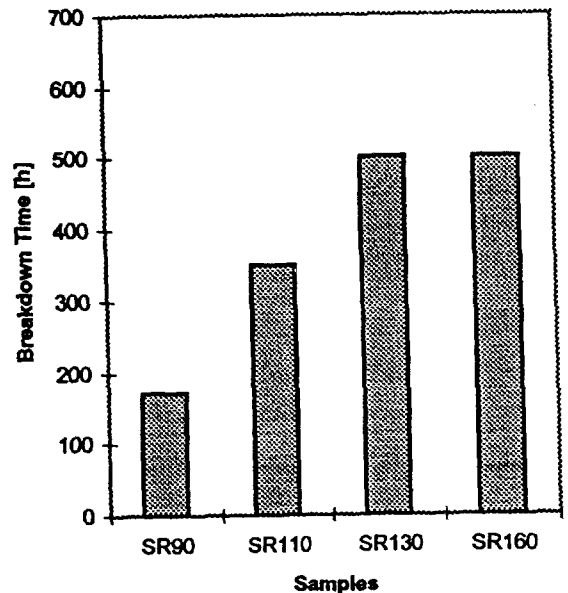
그림 10. 시료에 대한 절연 파괴 시간 Fig. 10. Failure time for samples
