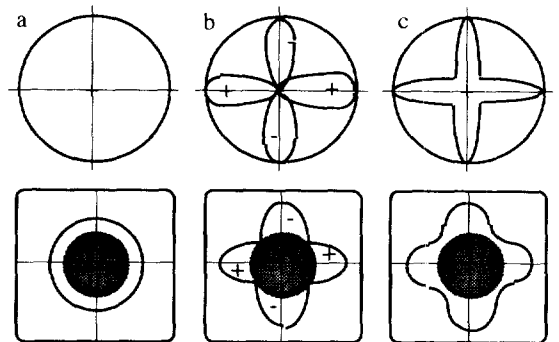
그림 2. a. isotropic s-wave b. d-wave c. anisotropic s wave
