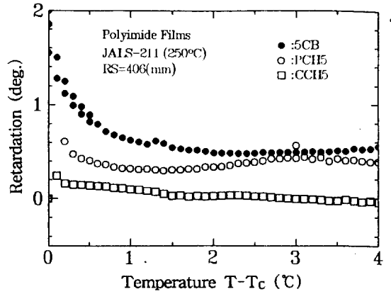
그림 7. 강하게 러빙처리된 폴리이미드막에 있어서 분자구조가 다른 3종류의 네마틱액정에 관한 상전이온도 이상의 온도영역에 있어서의 잔류광학 리타레이션의 온도의 존성.
