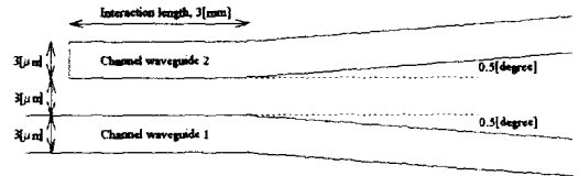
그림 2. 광결합기의 구조 Fig. 2. Structure of optical coupler.
