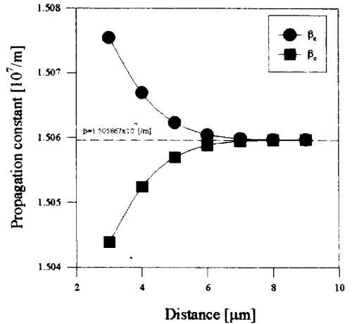
그림 4. 채널도파로 간격에 따른 대칭모드와 비대칭모드의 전파상수
