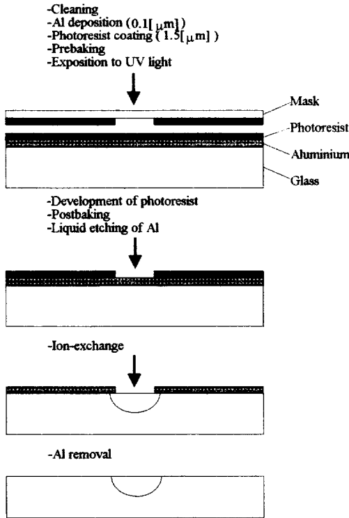
그림 3. 채널도파로 제작공정도
