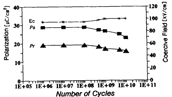
그림 5. 47/53 PZT 박막의 피로도
