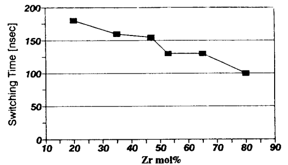
그림 7. Zr/Ti 비에 따른 스위칭 시간의 변화
