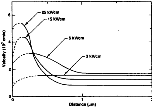
그림 3. 캐리어의 과도 현상
