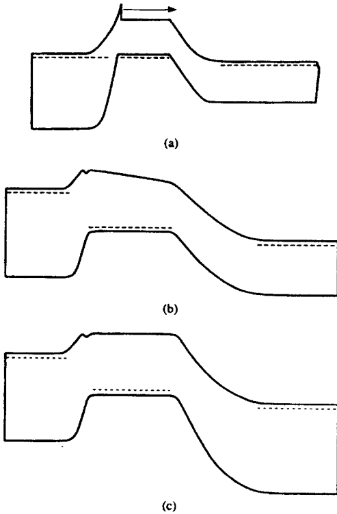
그림 4. 에너지대역에 의한 HBT의 종류
