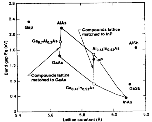
그림 2. 에너지 대역 간극과 격자 상수
