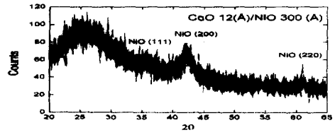
그림 8-(a). CoO 12A /NiO 300A 박막의 XRD data.
