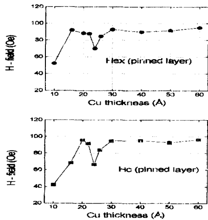
그림 4. NiO 400Å /NiFe 60Å /Cu 10Å ~60Å/NiFe 60Å 박막에서 pinned layer의 교환력과 보자력.
