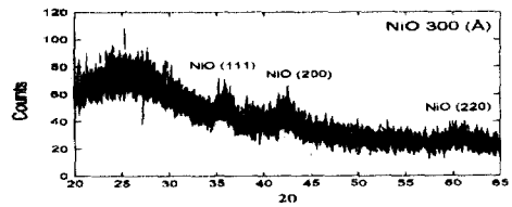
그림 8-(b). NiO 300A 박막의 XRD data.
