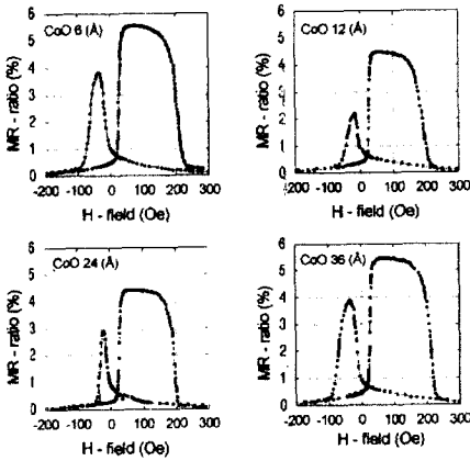
그림 5. \text{CoO}_{6\text{Å}}\text{-}_{360\text{Å}}/\text{NiO}_{400\text{Å}}/\text{NiFe}_{60\text{Å}}/\text{Cu}_{16\text{Å}}/\text{NiFe}_{60\text{Å}} 박막의 자기저항 곡선.
