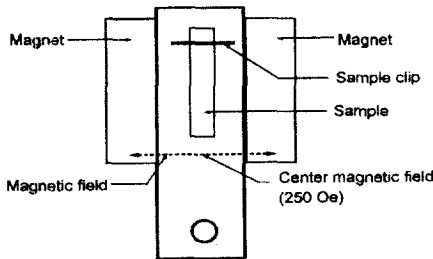
그림 1. 시료 장착 구조도
