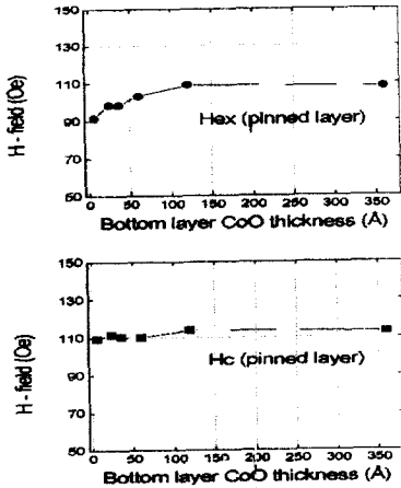
그림 6. \text{CoO}_{6\text{Å}}\text{-}_{360\text{Å}}/\text{NiO}_{400\text{Å}}/\text{NiFe}_{60\text{Å}}/\text{Cu}_{16\text{Å}}/\text{NiFe}_{60\text{Å}} 박막에서 pinned layer의 교환력과 보자력.
