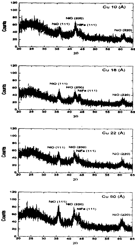
그림 7. NiO 40A /NiFe 40A /Cu 10A~50A /NiFe 40A 박막의 XRD data.
