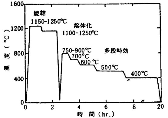
그림 5. Sm 2 (Co, Fe, Cu, Zr) 17 계 자석에 관한 다량 시효와 소결의 모식도
