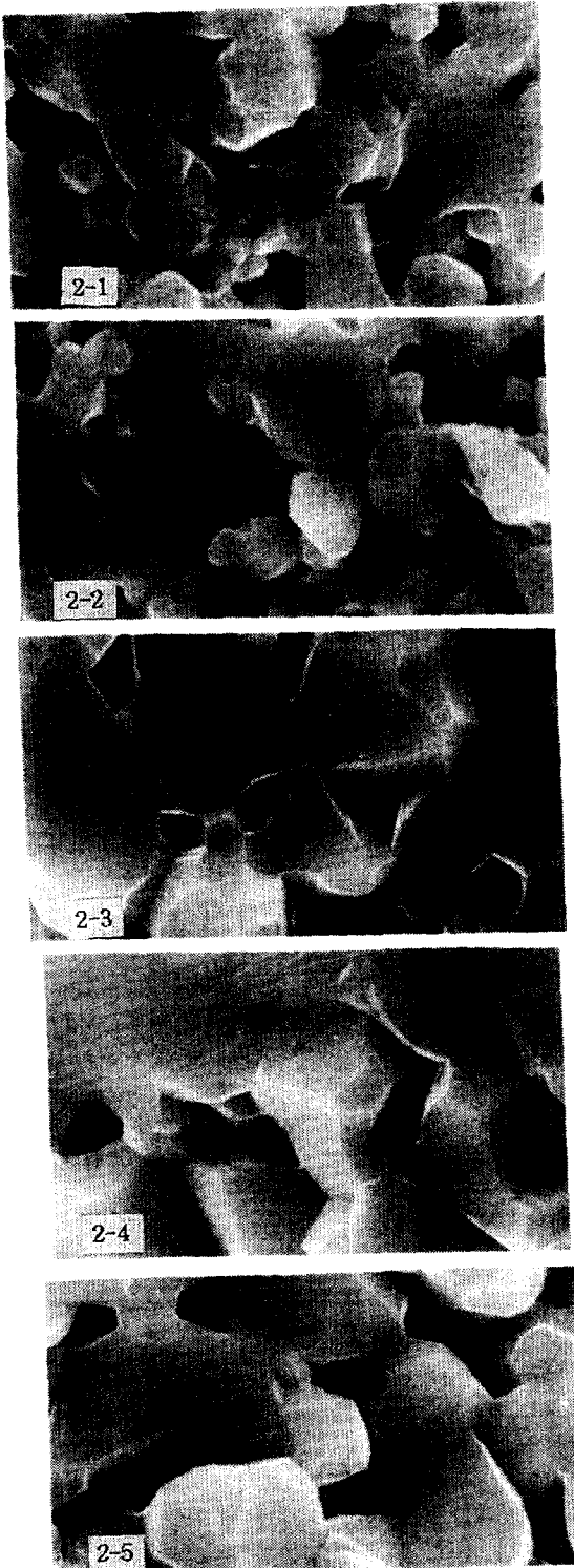
그림 3-3. NiO의 양에 따른 SEM사진( \times 8,000 ) Fig. 3-3. SEM micrographs according to NiO contents( \times 8,000 ).
