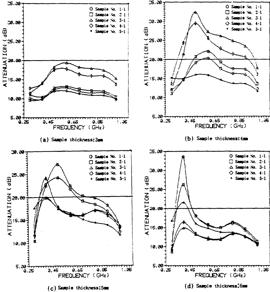
그림 3-6. Ni-Zn페라이트의 감쇄량에 따른 주파수 의존성
