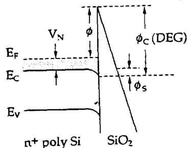
(b) 축퇴된 다결정 실리콘 (b) De generated poly-silicon
