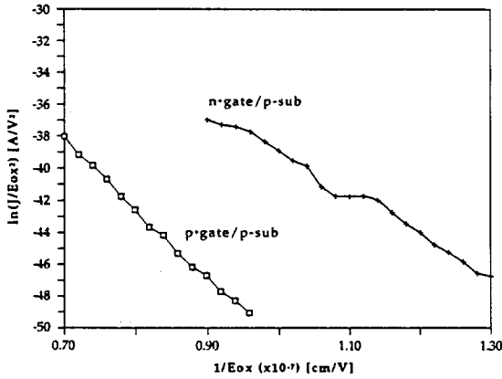
그림 4. 게이트 전극에 따른 \ln(J/E_{ox}^2) - 1/E_{ox} 특성
