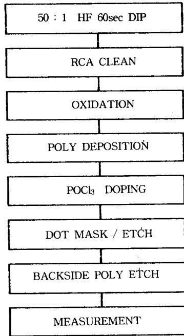
그림 3. MOS캐패시터 제작의 공정 순서도 Fig. 3. Process flowchart for MOS capacitor fabrication
