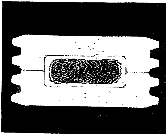
그림 6. Furukawa 전공에서 개발한 Cluster Back-Up 코일용 도체 단면
