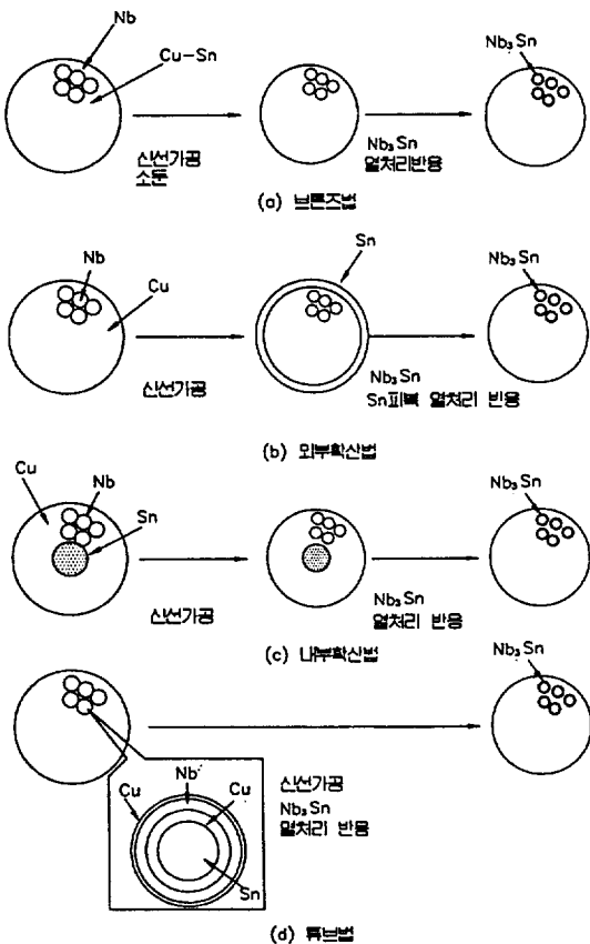
그림 2. Nb 3 Sn초전도선재, 도체제조를 위한 브론즈법과 개량브론즈법
