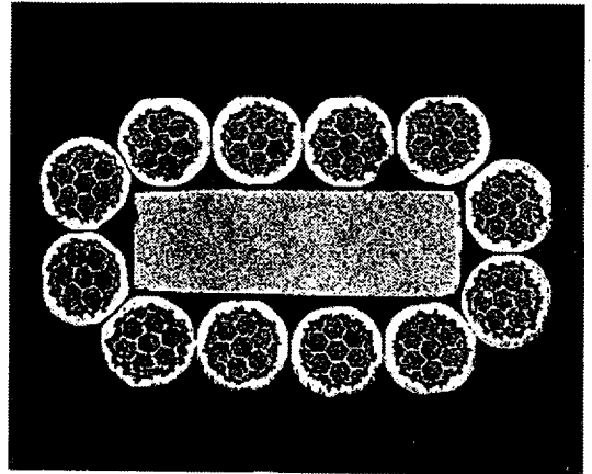
그림 7. Furukawa 전공에서 개발한 초전도발전기 계자코일용 Nb 3 Sn 집합도체의 단면
