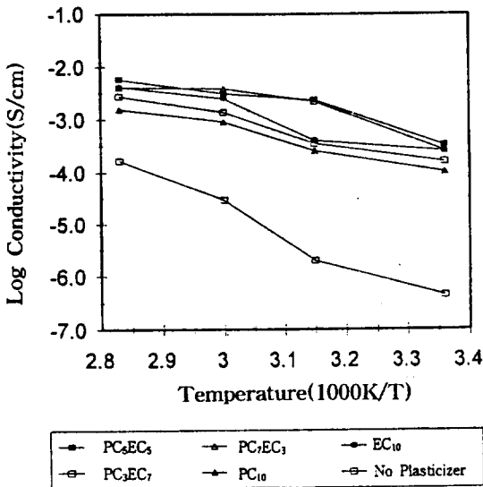
그림 6. 가소제 첨가에 따른 \text{PEO}_8\text{LiClO}_4 전해질 필름의 전도도 변화. Fig. 6. Variation of conductivity of \text{PEO}_8\text{LiClO}_4 electrolyte film by plasticizer addition.
