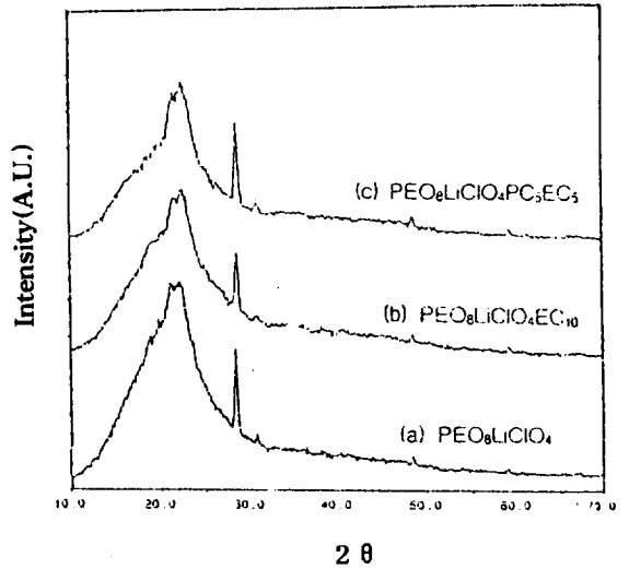
그림 7. 가소제 첨가에 따른 \text{PEO}_8\text{LiClO}_4 전해질 필름의 X-선 회절 패턴의 변화. Fig. 7. Change of X-ray diffraction patterns of \text{PEO}_8\text{LiClO}_4 electrolyte film by plasticizer addition.
