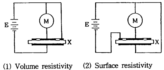
그림. 4. 체적고유 저항 및 표면고유 저항을 측정 회로.
