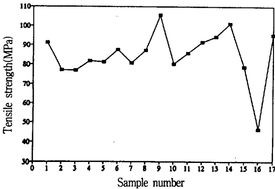
그림. 2. 시작품의 인장강도 특성.
