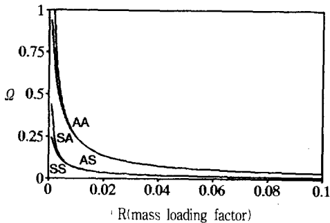
그림 10. s-1의 질량부하에 대한 기준각주파수
