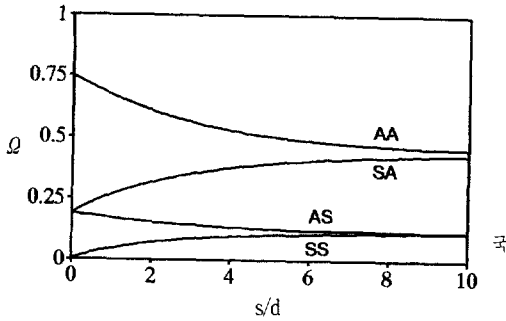
그림 7. s-4의 비전극부분의 폭과 세라믹의 두께비에 대한 기준각주파수.
