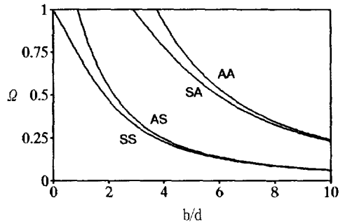
그림 8. s-1의 전극부분의 폭과 세라믹의 두께비에 대한 기준각주파수
