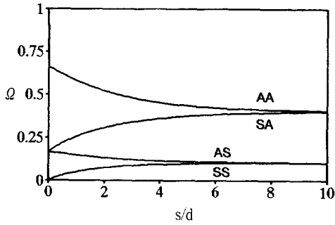
그림 6. s-1의 비전극부분의 폭과 세라믹의 두께비에 대한 기준각주파수
