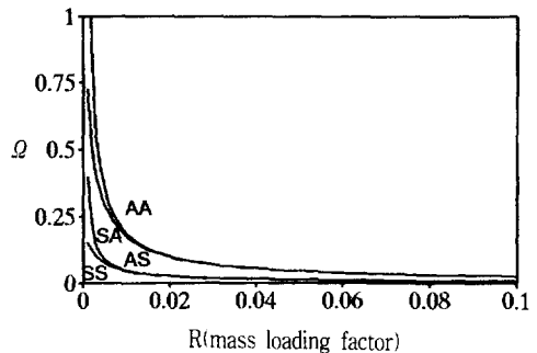
그림 11. s-4의 질량부하에 대한 기준각주파수
