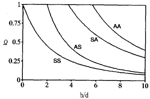
그림 9. s-4의 전극부분의 폭과 세라믹의 두께비에 대한 기준각주파수.
