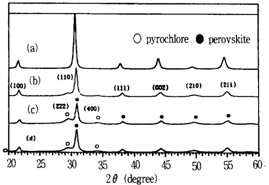
그림 10. 촉매의 첨가에 따른 PZT(x=0.575) 분말의 XRD 패턴: (a) 질산촉매, (b) 4시간 열처리에 따른 암모니아수 촉매 (c) 30분 열처리에 따른 암모니아수 촉매, (d) 무촉매
