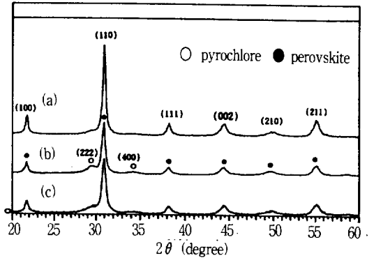
그림 9. 촉매의 첨가에 따른 PZT(x=0.535) 분말의 XRD 패턴:(a) 질산촉매, (b) 무촉매, (c) 암모니아수 촉매
