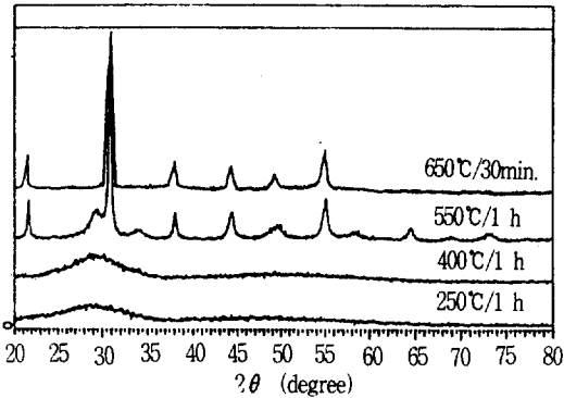
그림 7. 각 온도에서 열처리한 PZT 분말의 XRD 패턴(촉매:질산)
