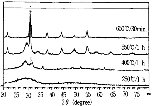
그림 8. 각 온도에서 열처리한 PZT 분말의 XRD 패턴(촉매:암모니아수)
