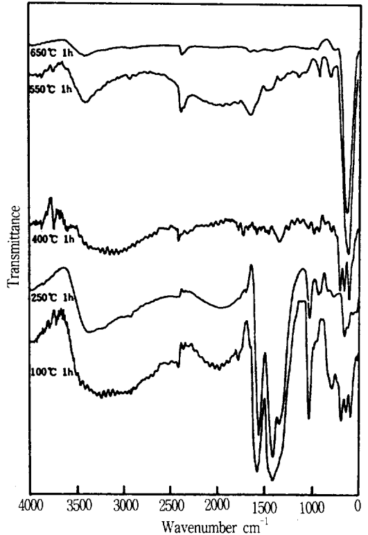
그림 4. 질산을 이용하여 제조된 젤의 적외선 분광 분석 Fig. 4. FT-IR spectra of gel prepared by using HNO 3 .
