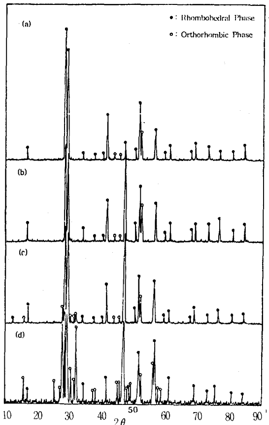
그림 2. 소결한 PbNb_2O_6 분말의 X선 회절분석
