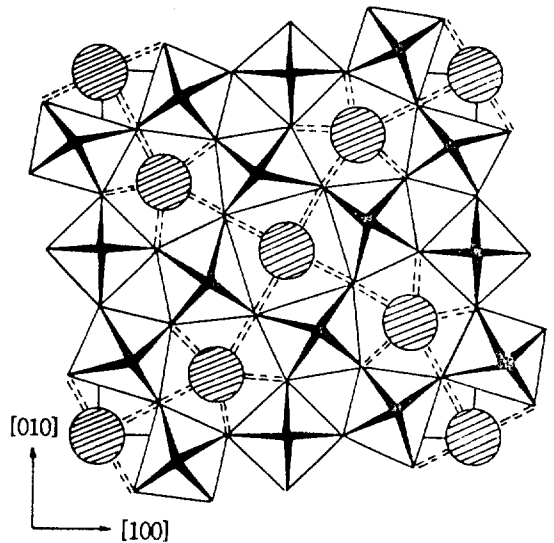
그림 4. [001]방향에 평행한 상유전 PbNb 2 O 6 의 구조 6)
