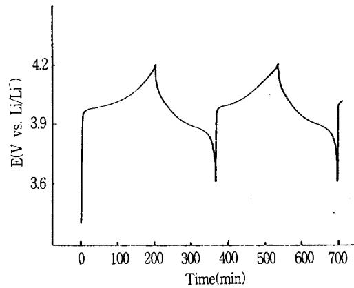
그림 7. CFM-LiCoO 2 /Li 전지의 정전류충방전 특성. 충방전 전압범위 ; 3.6V~4.2V 전류밀도 ; 1mA/cm 2
