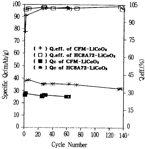
그림 6. 순환전압-전류법에 의한 CFM-LiCoO 2 및 HC8A72-LiCoO 2 의 비환원용량 및 산화환원 효율의 변화. 전위영역 ; 3.6V~4.2V 주사속도 ; 0.5mV/sec Fig. 6. Variation of the cathodic specific capacity and Q.eff. of CFM-LiCoO 2 and HC8A72-LiCoO 2 during CV. potential range ; 3.6V~4.2V. scan rate ; 0.5mV/sec
