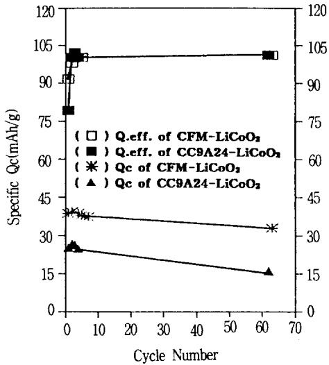
그림 4. 순환전압-전류법에 의한 CFM-LiCoO 2 및 CC9A24-LiCoO 2 의 비환원용량 및 산화-환원 효율의 변화. 전위영역 ; 3.0~4.5V 주사속도 ; 2mV/sec
