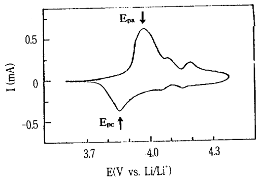
그림 2. CFM-LiCoO 2 전극의 순환전압전류그림 전위영역; 3.6V~4.4V 주사속도; 0.01mV/sec Fig. 2. Cyclic voltammogram for CFM-LiCoO 2 electrode. potential range ; 3.6V~4.4V scan rate ; 0.01mV/sec
