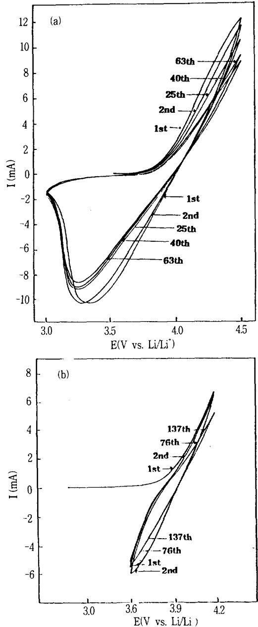
그림 3. 주사속도 및 전위영역 변화에 따른 CFM-LiCoO 2 전극의 순환전압전류그림. 전위영역 ; (a) 3.0~4.5V, (b) 3.6~4.2V 주사속도 ; (a) 2mV/sec, (b) 1mV/sec
