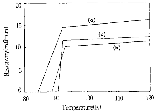
그림 1. PLD법에 의해 제작된 YBa 2 Cu 3 O 7-x 초전도체 박막의 R-T 곡선: (a) P O2 =0, T sub =650°C, 분위기로 열처리, (b) P O2 =200 mTorr, T sub =750°C, 분위기로 열처리, (c) P O2 =200mTorr, T sub =750°C, in-situ 열처리
