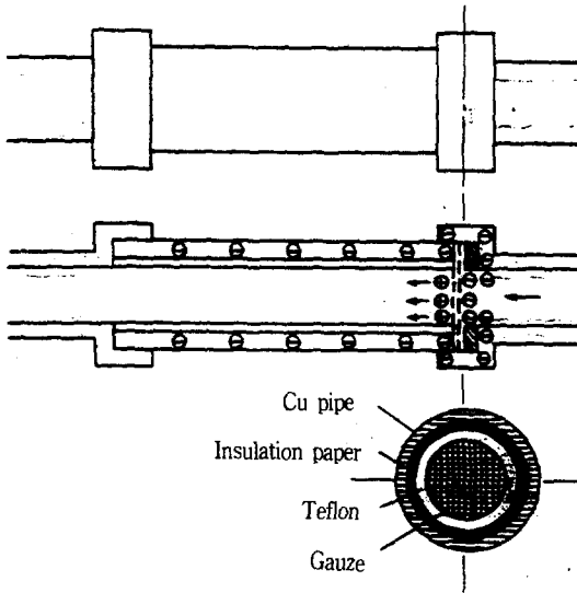
그림 2 가제 대전장치 개략도 Fig. 2 Diagram of gauze electrification apparatus.
