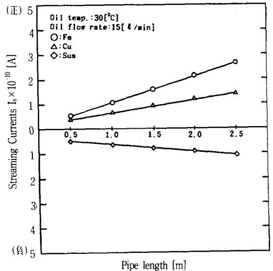
그림 9 유동전류의 파이프길이 의존성
