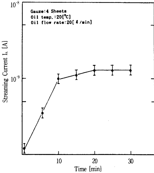
그림 4 유동전류의 시간 의존성 Fig. 4 Dependence of streaming currents on oil temp.
