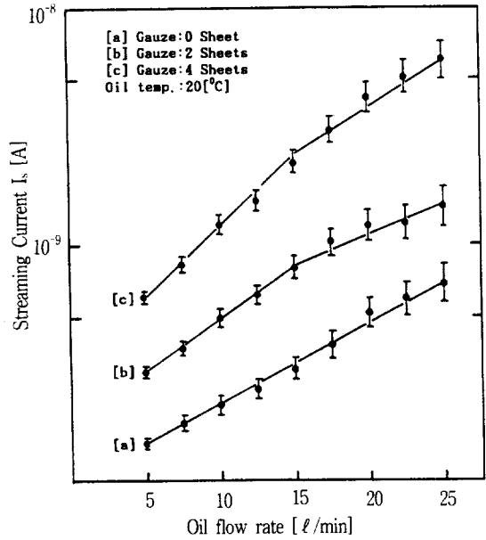
그림 5 유동전류의 유량 의존성 Fig. 5 Dependence of streaming currents on flow rate.
