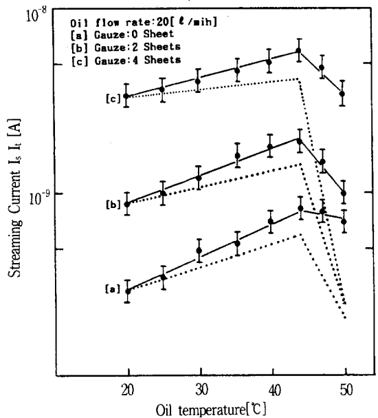
그림 6 유동전류의 유온 의존성 Fig. 6 Dependence of streaming currents on oil temp.
