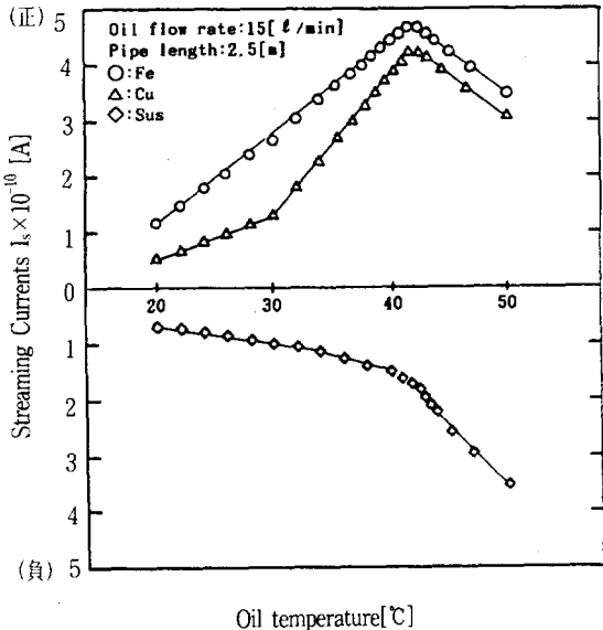
그림 7 유동전류의 유온 의존성
