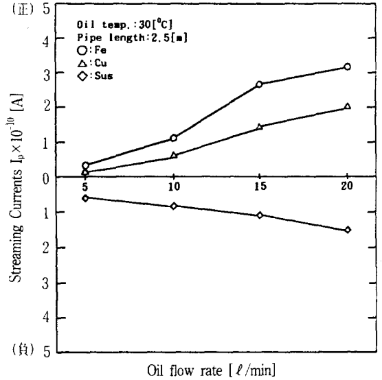
그림 8 유동전류의 유량 의존성
