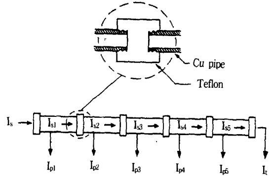
그림 3 파이프 대전장치 개략도 Fig. 3 Diagram of pipe electrification apparatus.
