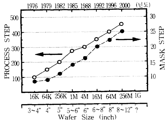
그림 2 DRAM대용량화에 따른 공정수와 mask수의 증가추이
