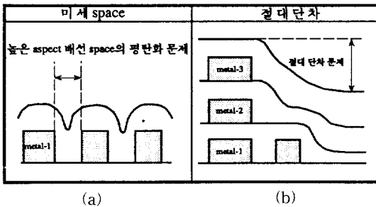
그림 7 배선 층간막 평탄화 기술문제
