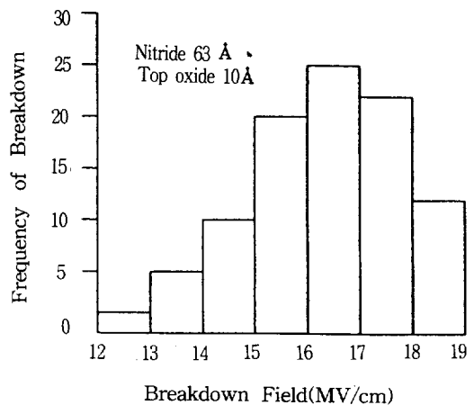
그림 8 상층산화막의 두께를 파라미터로 한 MONOS 축전기의 절연파괴 강도
