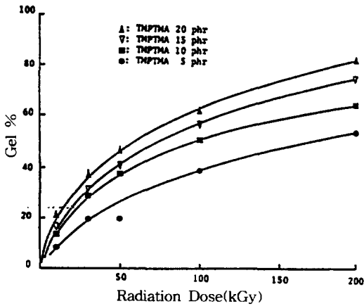
그림 2 TMPTMA의 양과 조사선량에 따른 가교도(gel %)
