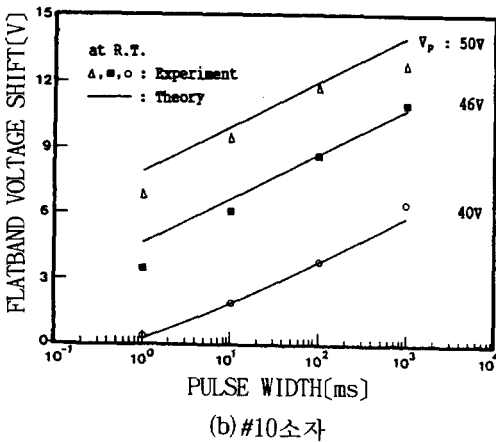
그림 5 t_p 에 대한 \Delta V_{FB} 특성의 이론치와 실험치의 비교 (#53, #10소자) Fig. 5 Characteristics of the t_p versus \Delta V_{FB} comparison between experimental and theoretical values, (#53, #10 device)
