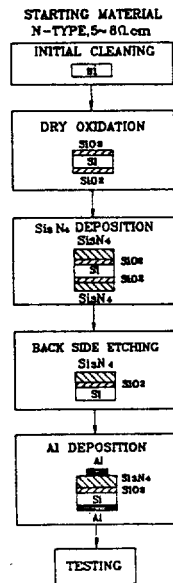
그림 2 MNOS소자의 구조 및 제작과정 Fig. 2 Process sequence and cross section of MNOS fabrication.
