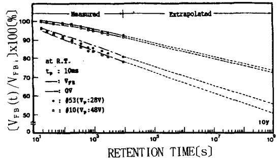
그림 10 포획전하의 유지조건에 따른 기억 유지특성 (#53, #10소자) Fig. 10 Retention characteristics at V_{FB} and zero voltage bias, (#53, #10 device)
