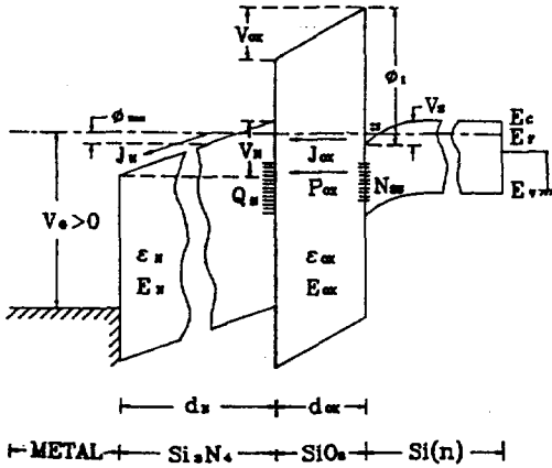
그림 1. 양의 게이트 전압 인가시 에너지밴드 다이어그램과 전하주입과정 Fig. 1 Energy band diagram and charge injection process under positive bias.
