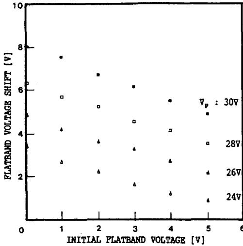
그림 9 펄스전압에 따른 초기 플랫밴드전압 변화의 기울기 (#53소자) Fig. 9 The slope of \Delta V_{FB} versus V_{FB0} with pulse amplitude, (#53 device)
