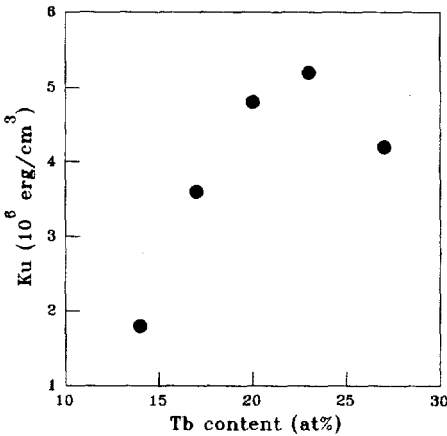
그림 6. Tb_x(Fe_{0.9}Co_{0.1})_{100-x} 시료의 Tb 함량에 따른 수직 자기이방성계수 Fig. 6 Compositional dependence of perpendicular anisotropy K_u at room temperature for Tb_x(Fe_{0.9}Co_{0.1})_{100-x} specimen films.
