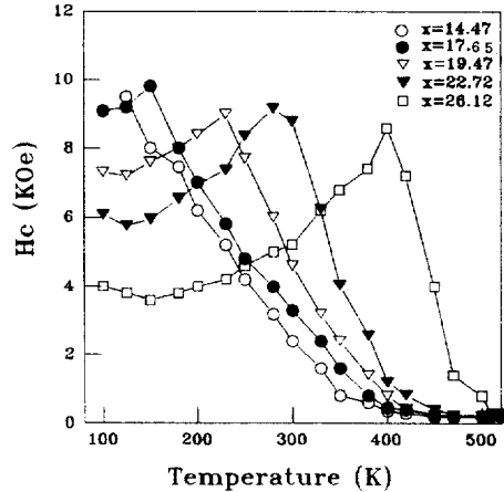
그림 5. Tb_x(Fe_{0.9}Co_{0.1})_{100-x} 시료의 조성별 보자력의 온도 의존성
