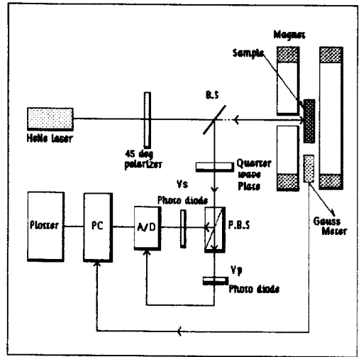
그림 2. Polar Kerr각 이력곡선 측정장치 Fig. 2. Experimental set-up for polar Kerr angle hysteresis loop measurement.
