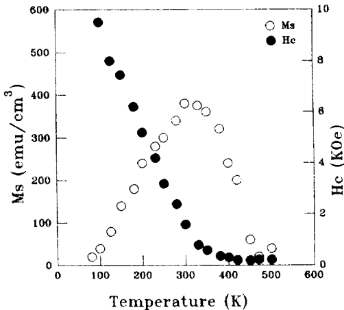
그림 4. Tb_{14.47}(Fe_{77.84}Co_{7.69}) 시료의 포화자화 및 보자력의 온도 의존성
