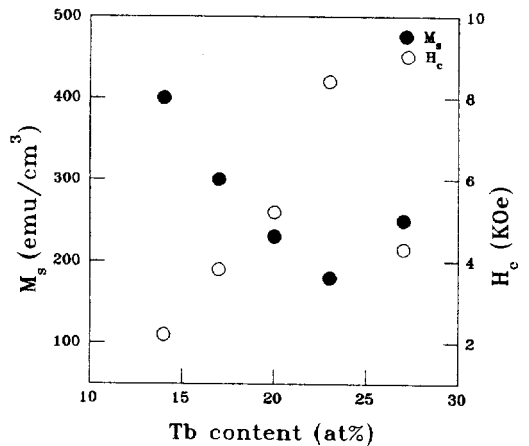
그림 3. Tb_x(Fe_{0.9}Co_{0.1})_{100-x} 시료의 Tb 함량에 따른 포화자화 및 보자력 Fig. 3. Compositional dependence of saturation magnetization and coercivity at room temperature Tb_x(Fe_{0.9}Co_{0.1})_{100-x} specimen films
