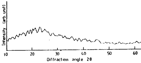
그림 1. Tb_{26.12}(Fe_{63.53}Co_{10.7}) 시료의 X-선 회절 패턴 Fig. 1. X-ray diffraction pattern of Tb_{26.12}(Fe_{63.53}Co_{10.7}) specimen film.
