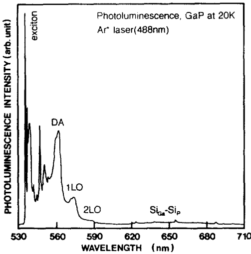
그림8. 20K 온도에서 측정된 GaP의 광루미네선스 스펙트럼. Fig.8. Photoluminescence spectrum of GaP measured at 20K.
