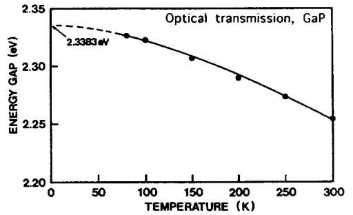
그림7. 광투과방법으로 측정한 에너지갭의 온도의존성.
