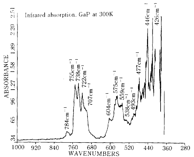
그림11. 300K의 온도에서 측정된 GaP의 적외선 흡수스펙트럼. Fig.11. Infrared absorption spectrum of GaP at 300K.
