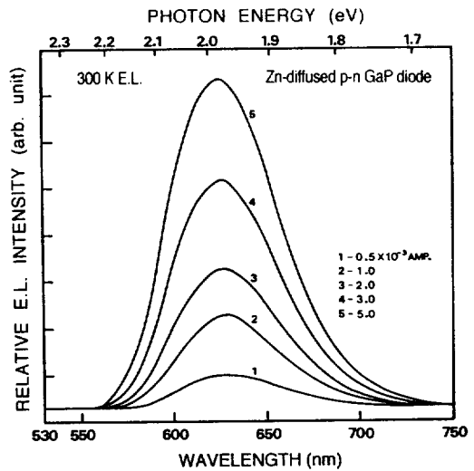
그림12. Zn를 확산시켜 제작한 GaP발광다이오드의 주입전류에 따른 전계루미네선스 스펙트럼.(300K)
