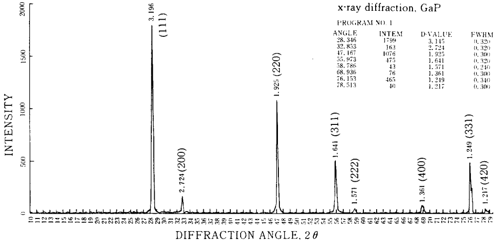
그림5. GaP결정의 x선 회절도.
