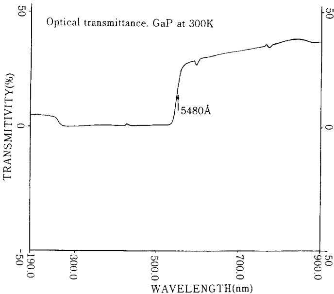
그림6. 300K 온도에서 측정된 GaP의 광투과도.
