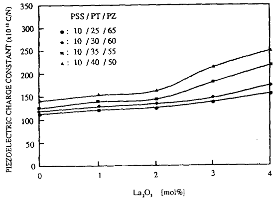
그림 3-5. 0, 10PSS-xPT-(0, 90-x)PZ시편의 La 2 O 3 첨가량에 따른 압전전하계수
