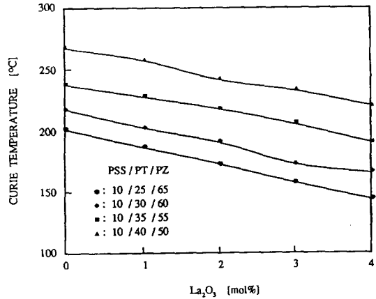
그림 3-4. 0, 10PSS-xPT-(0, 90-x)PZ시편의 La 2 O 3 첨가량에 따른 큐리온도 Fig. 3-4. Curie temperature with contents of La 2 O 3 in the 0, 10PSS-xPT-(0, 90-x)PZ specimens.
