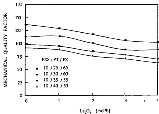
그림 3-7. 0.10PSS-xPT-(0.90-x)PZ시편의 \text{La}_2\text{O}_3 첨가량에 따른 기계적 품질계수
