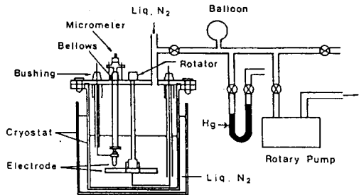
그림 1. 실험장치의 개략도
