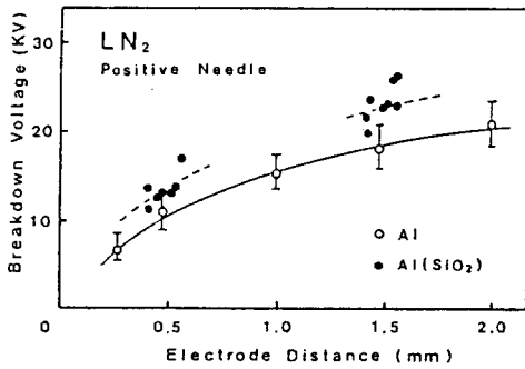
그림 10. 액체 N 2 파괴특성의 전극피복효과 Fig.10. Coating effect of electrode in Liq. N 2 .
