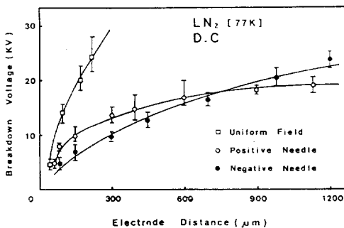
그림 6. 액체 N 2 의 절연파괴전압의 극성별 전극간 거리의존성 Fig.6. Dependence of electrode distance in Liq.N 2 .
