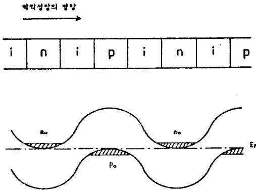
그림 3. nipi초격자의 구조와 에너지대. 주기적으로 도우핑을 행함으로써 퍼텐셜에너지도 주기적으로 변화시킬 수 있다. 단 전자, 양공은 공간적으로 분리되어 있다.
