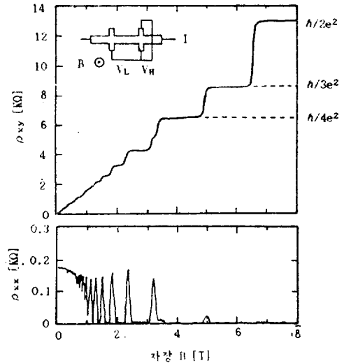
그림 13. 선택도우프한 GaAs/AlGaAs 초격자의 50mK에서의 전류방향의 저항률 \rho_{xx} 와 전류에 수직방향의 저항률(Hall 저항률) \rho_{xy} 에서 관측된 양자 Hall 효과 8) . \rho_{xy} 는 계단상으로 되어 있는데 평탄한 부분의 값은 h/e^2 의 정수분의 1로 되어 있다. \rho_{xx} 의 평탄한 부분에 대응하여 \rho_{xx} 는 0으로 되어 있다.
