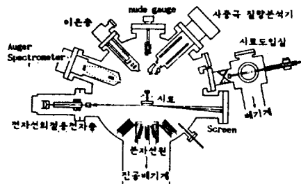
그림 6. MBE장치의 개략도
