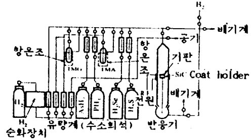
그림 7. MOCVD장치의 개략도
