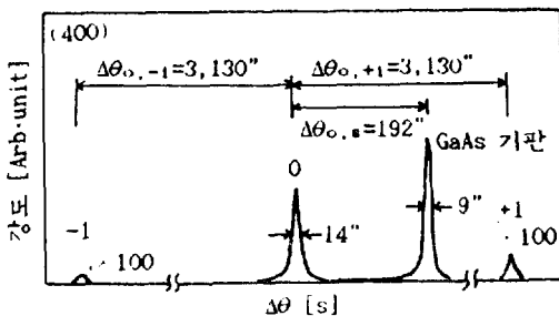
그림 8. 2결정법에 의한 GaAs/AlAs 초격자의 X선회절패턴 2)
