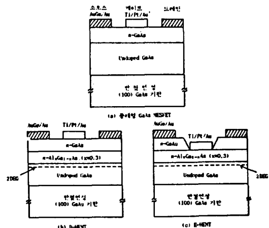
그림 14. 각종 GaAs계 전계효과 트랜지스터의 구조 비교.
