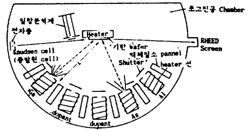
그림 5. MBE성장의 원리도
