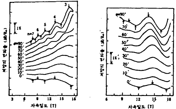
(b) AlGaAs 장벽층이 상당히 두꺼워 (90Å), 전자가 (90°) 양자우물내에 완전히 갇혀져 있는 경우
