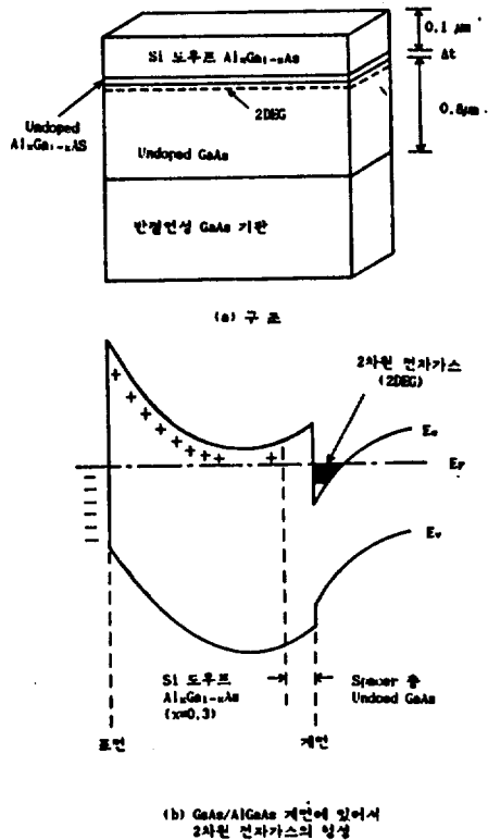
그림 12. 변조도우프 초격자구조에 의한 2차원 전자가스의 형성과 이온화불순물산란의 제거
