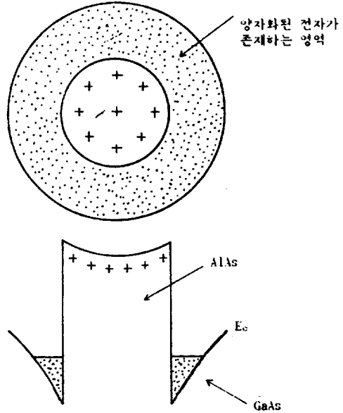
그림 18. Superatom의 구조
