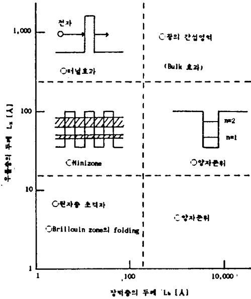
그림 4. 장벽층의 두께 L_b , 우물층의 두께 L_s 과 초격자의 전자적, 광학적 성질의 관계
