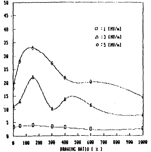
그림 10. 연신비에 따른 열자극전류의 피크값 Fig. 10. Peak value of TSC with draw ratio.
