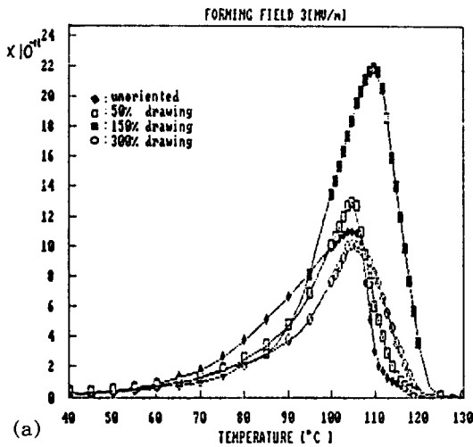
그림 4. 인장비에 따른 열자극전류의 온도의존성 (E=3(MV/m)) Fig. 4. Temperature dependence of TSC due to variation of draw ratio (E=3(MV/m)).
