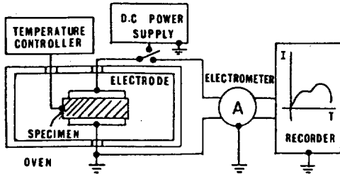
그림 2. 열자극전류 실험장치의 블럭선도 Fig 2. Block diagram of TSC apparatus.
