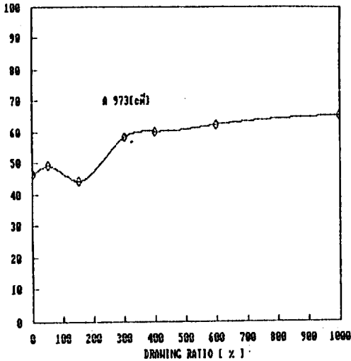
그림 8. 연신비에 따른 적외선 흡수량 (973(cm -1 ))
