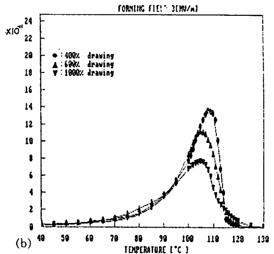
그림 4. 인장비에 따른 열자극전류의 온도의존성 (E=3(MV/m)) Fig. 4. Temperature dependence of TSC due to variation of draw ratio (E=3(MV/m)).
