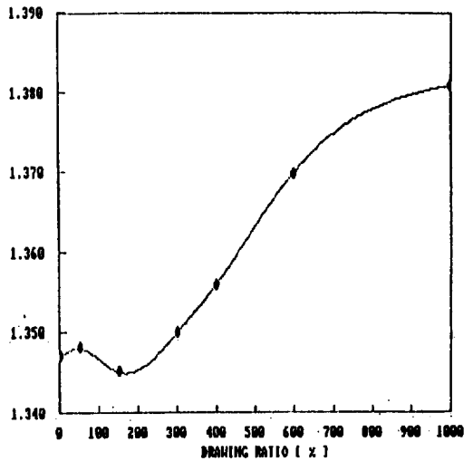
그림 9. 연신비에 따른 밀도 변화
