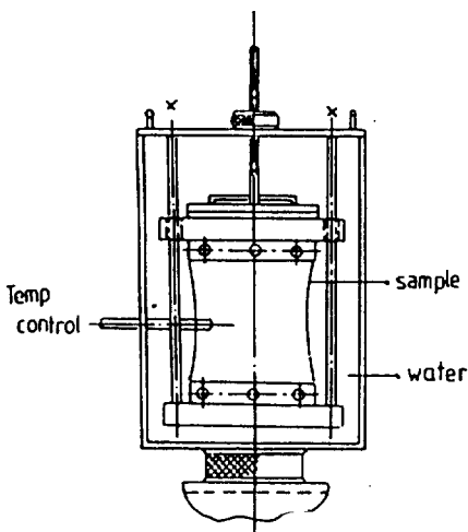
그림 1. 시료의 연신장치
