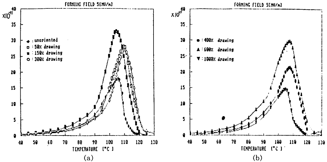
그림 5. 인장비에 따른 열자극전류의 온도의존성 (E=5(MV/m))
