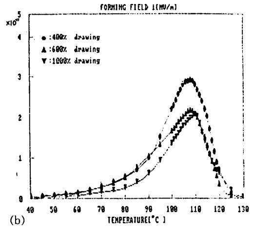
그림 3. 인장비에 따른 열자극전류의 온도의존성 (E=1(MV/m)) Fig. 3. Temperature dependence of TSC due to variation of draw ratio (E=1(MV/m)).
