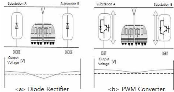
Fig. 2. Diode rectifier and PWM converter. (a) Diode rectifier. (b) PWM converter.
