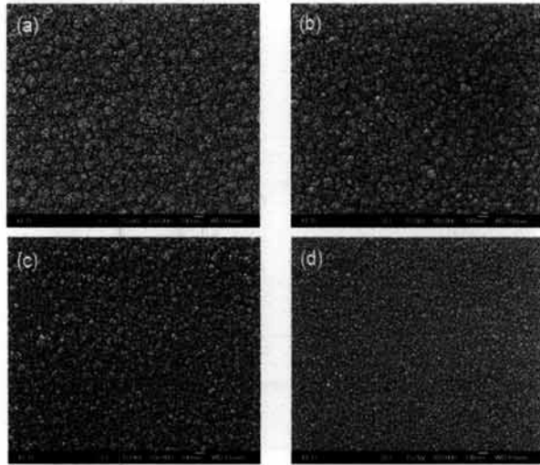
Fig. 3. SEM analysis of (SiO_2)_x-(Ti)_y MDTF surface, (a) (SiO_2)_{90}-(Ti)_{10} , (b) (SiO_2)_{80}-(Ti)_{20} , (c) (SiO_2)_{70}-(Ti)_{30} , (d) (SiO_2)_{60}-(Ti)_{40} .
