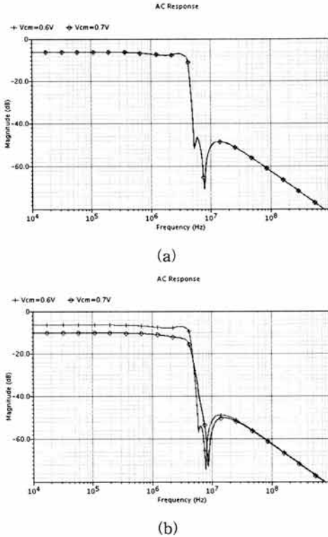
그림 8. 입력 공통 모드 전압 변화에 따른 Gm-C LPF 주파수 특성: (a) CMFF 있을 때, (b) CMFF 없을 때.
