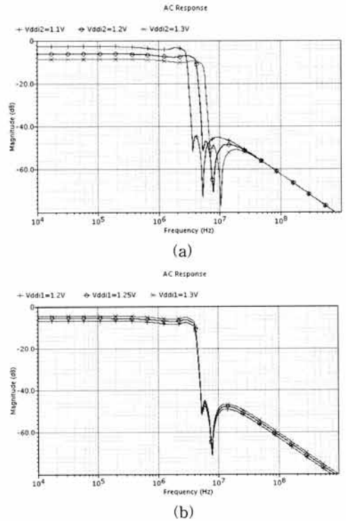
그림 7. Gm-C LPF 주파수 특성: (a) 주파수 튜닝, (b) 이득 튜닝.
