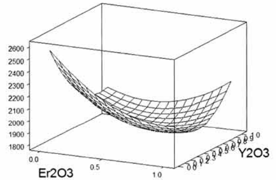
그림 3. Y 2 O 3 및 Er 2 O 3 첨가량에 따른 유전율. Fig. 3. Dielectric constant as a function of content of Y 2 O 3 and Er 2 O 3 .
