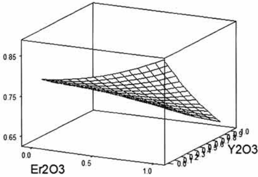
그림 4. Y_2O_3 및 Er_2O_3 첨가량에 따른 유전손실. Fig. 4. Dielectric loss as a function of content of Y_2O_3 and Er_2O_3 .
