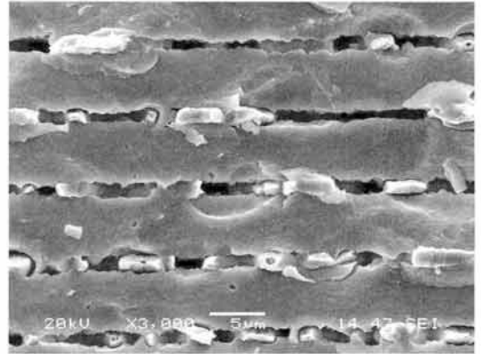
그림 8. MLCC의 내부 단면구조.
