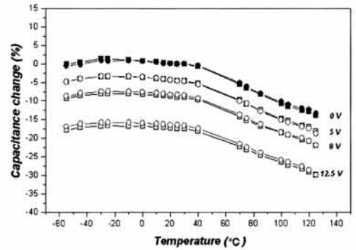
그림 9. 온도 및 인가전압 변화에 따른 용량 특성.
