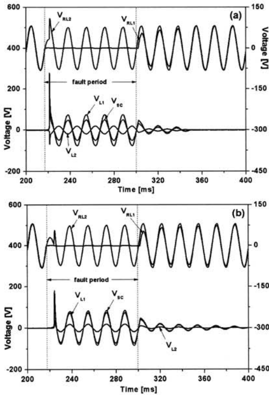
그림 5. 병렬연결된 두 코일의 자기결합을 이용한 초전도 전류제한기의 전압강하 보상특성. (a) 가극결선시 (b) 감극결선시.
