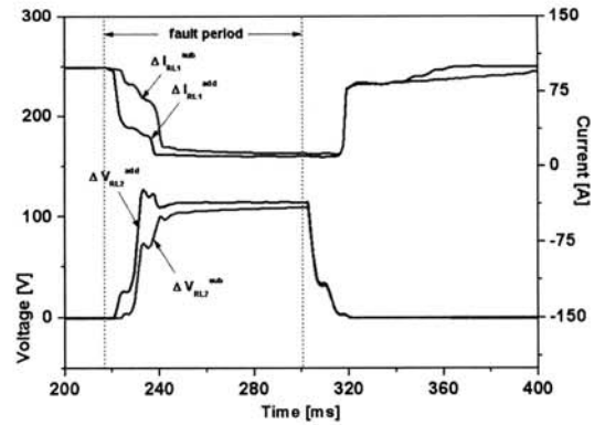
그림 6. 병렬연결된 두 코일의 자기결합을 이용한 초전도 전류제한기의 부하전압강하율 및 전류제한율을 변화.
