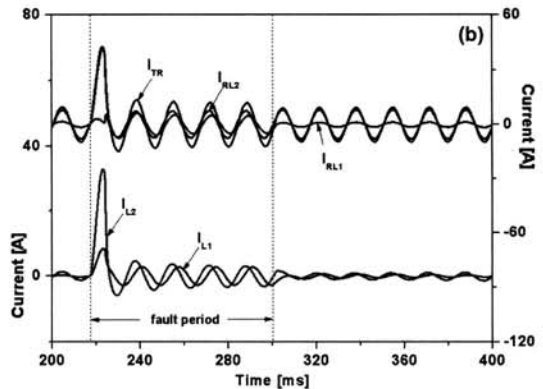
그림 4. 병렬연결된 두 코일의 자기결합을 이용한 초전도 전류제한기의 전류제한 특성. (a) 가극결선시 (b) 감극결선시
