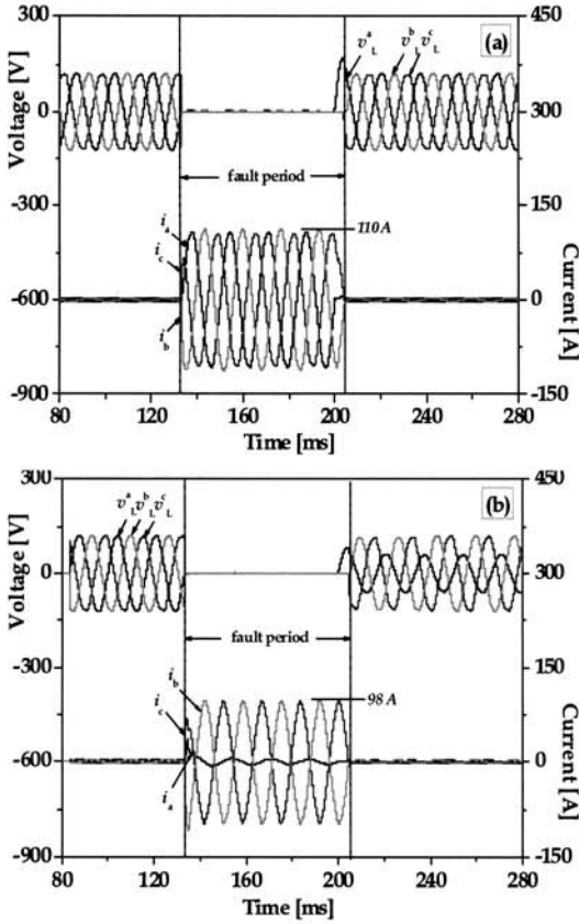
그림 5. 삼선지락시 부하전압 및 선로전류. (a) 중성선에 초전도 전류제한기를 적용한 경우 (b) 중성선과 a상에 초전도 전류제한기를 적용한 경우 Fig. 5. Load voltages and line currents in case of the triple-line to ground fault. (a) a SFCL applied into neutral line (b) SFCLs applied into neutral line and a phase
