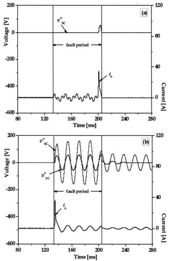
그림 6. 삼선지락시 초전도 전류제한기 전압 및 중성선 전류. (a) 중성선에 초전도 전류제한기를 적용한 경우 (b) 중성선과 a상에 초전도 전류제한기를 적용한 경우 Fig. 6. Voltage of SFCLs and neutral current in case of the triple-line to ground fault. (a) a SFCL applied into neutral line (b) SFCLs applied into neutral line and a phase
