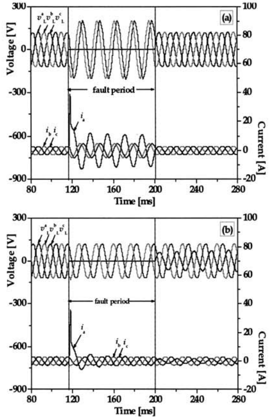
그림 2. 일선지락시 부하전압 및 선로전류. (a) 중성선에 초전도 전류제한기를 적용한 경우 (b) 중성선과 a상에 초전도 전류제한기를 적용한 경우
