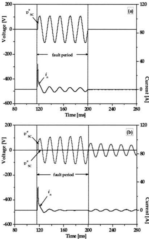
그림 3. 일선지락시 초전도 전류제한기 전압 및 중성선 전류.
