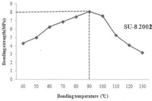
(a) 접합온도에 따른 SU-8의 접합강도
