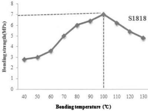
(a) 접합온도에 따른 S1818의 접합강도
