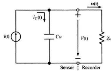
그림 3. 용량성 프로브의 등가회로. Fig. 3. Equivalent circuit of capacitive probe.
