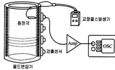
그림 6. 교정실험계의 구성.
