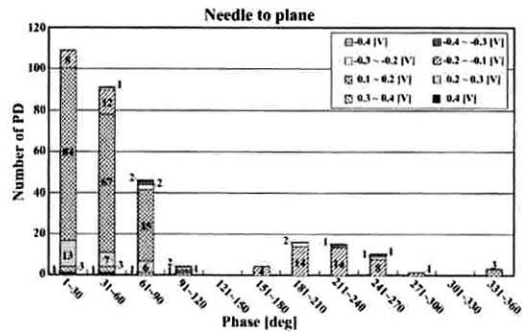
그림 11. \Phi -q-n 분석결과. Fig. 11. Result of \Phi -q-n analysis.
