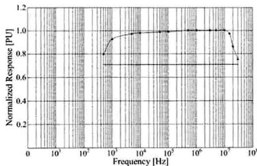
그림 5. 증폭회로의 주파수특성.
