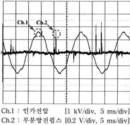
그림 9. 부분방전 펄스의 예. Fig. 9. Example of partial discharge pulses.
