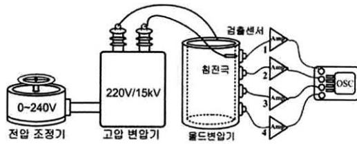
그림 12. 실험계의 구성.
