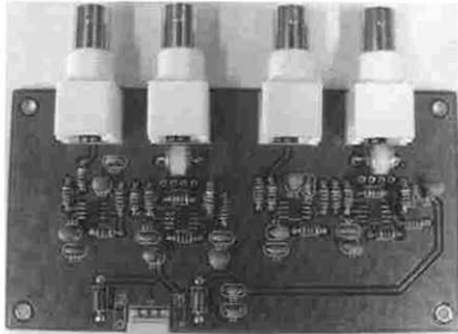
그림 4. 시제작 저잡음 증폭회로.
