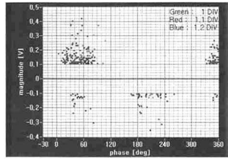
그림 10. 부분방전펄스의 위상분포. Fig. 10. Phase distribution of PD pulses.
