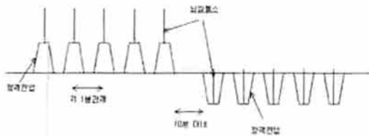
그림 2. 동작책무시험 패턴.
