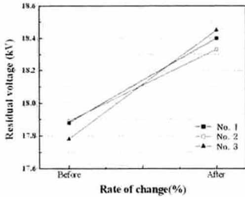
그림 5. 동작책무시험 전·후의 제한전압 변화. Fig. 5. Variation of residual voltage before and after operating duty test.
