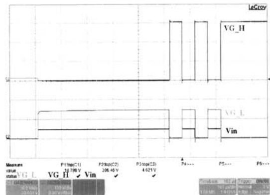
그림 8. 입력 및 출력 측정 파형. Fig. 8. The measured Input and output waveforms.
