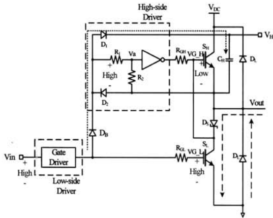
그림 2. Turn-off시 제안한 파워IC의 동작. Fig. 2. Operation of power IC at turn-off.
