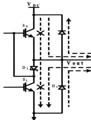
그림 1. 상단락 방지 구조의 half-bridge inverter. Fig. 1. Shoot-through immunity structure of half-bridge inverter.
