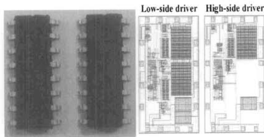
그림 6. 제작된 파워IC와 칩 레이아웃. Fig. 6. Package outline and chip layout of designed power IC.
