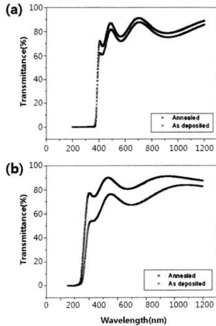
그림 3. (a) ZnO박막과 (b) GZO박막의 열처리 후 투과도 측정결과.
