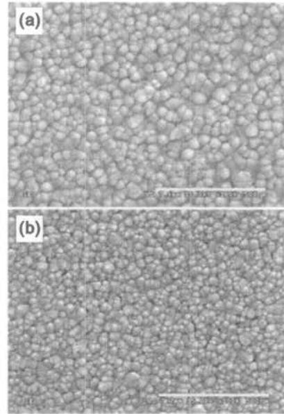
그림 1. (a) ZnO 와 (b) GZO 박막의 FE-SEM 이미지(scale bar : 500 nm).
