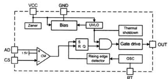
그림 1. 제안된 IC의 block diagram. Fig. 1. Block diagram of the proposed IC.
