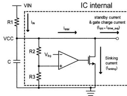
그림 2. IC의 내부 전원 bias의 구조도. Fig. 2. Internal scheme of voltage bias.
