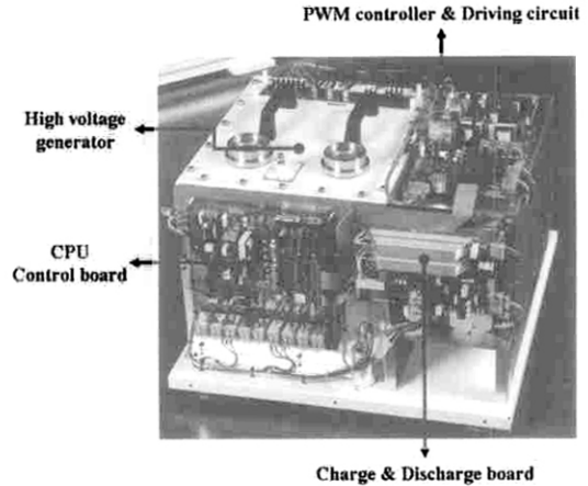
그림 2. 파워 유닛. Fig. 2. Power unit.
