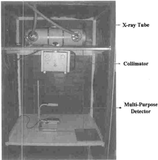
그림 5. 실험환경.
