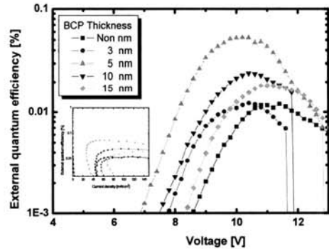
그림 7. BCP 두께변화에 따른 전압-외부양자효율.
