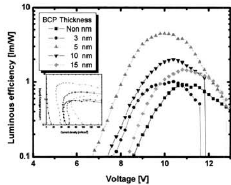
그림 6. BCP 두께변화에 따른 전압-발광효율.
