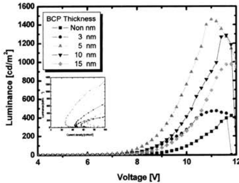
그림 5. BCP 두께변화에 따른 전압-휘도.
