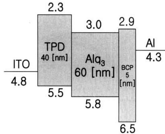
그림 3. BCP의 에너지 밴드. Fig. 3. Energy band of BCP.
