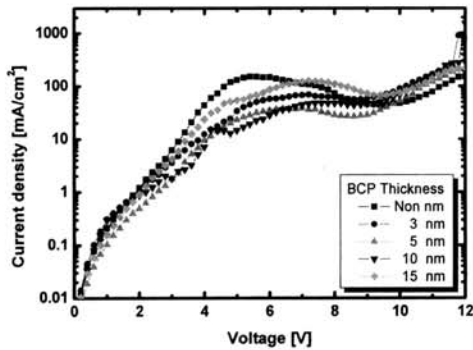
그림 4. BCP 두께변화에 따른 전압-전류밀도.
