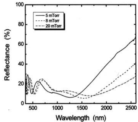
그림 9. 유리 기판 위에 증착된 ZnO:Al 박막의 스퍼터 압력에 따른 반사율.
