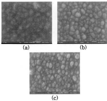
그림 3. 스퍼터 압력을 달리하여 PC 기판 위에 증착한 ZnO:Al 박막의 SEM 사진: (a) 2 mTorr; (b) 8 mTorr; (c) 20 mTorr.
