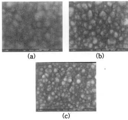
그림 4. PET 기판 위에 증착한 ZnO:Al 박막의 스퍼터 압력에 따른 SEM 사진: (a) 2 mTorr; (b) 8 mTorr; (c) 20 mTorr.
