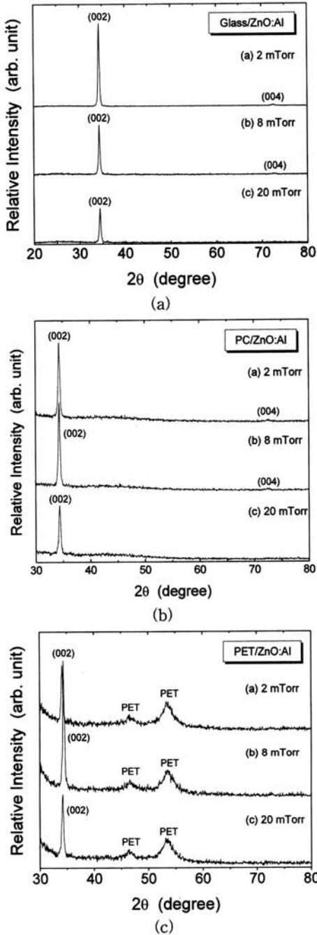
그림 2. ZnO:Al 박막의 스퍼터 압력에 따른 XRD pattern: (a) glass/ZnO:Al; (b) PC/ZnO:Al; (c) PET/ZnO:Al.
