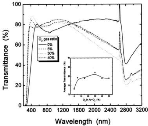
그림 1. 산소 가스 비에 따른 SnO 2 :Sb 박막의 광 투과율.
