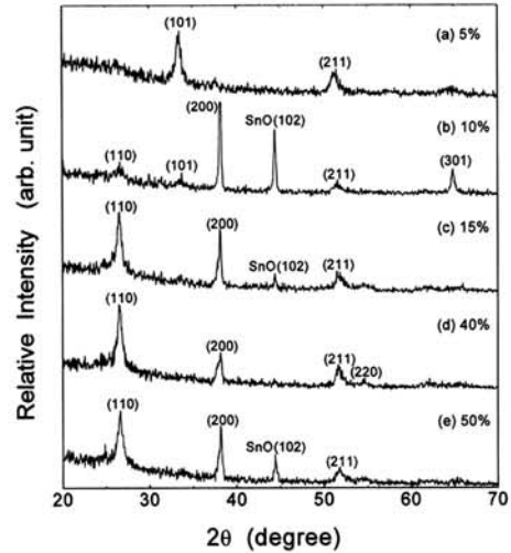
그림 2. 산소 가스 비에 따른 SnO 2 :Sb 박막의 XRD 패턴.
