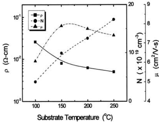
그림 6. SnO 2 :Sb 박막의 기판 온도에 따른 전기적 특성 변화.
