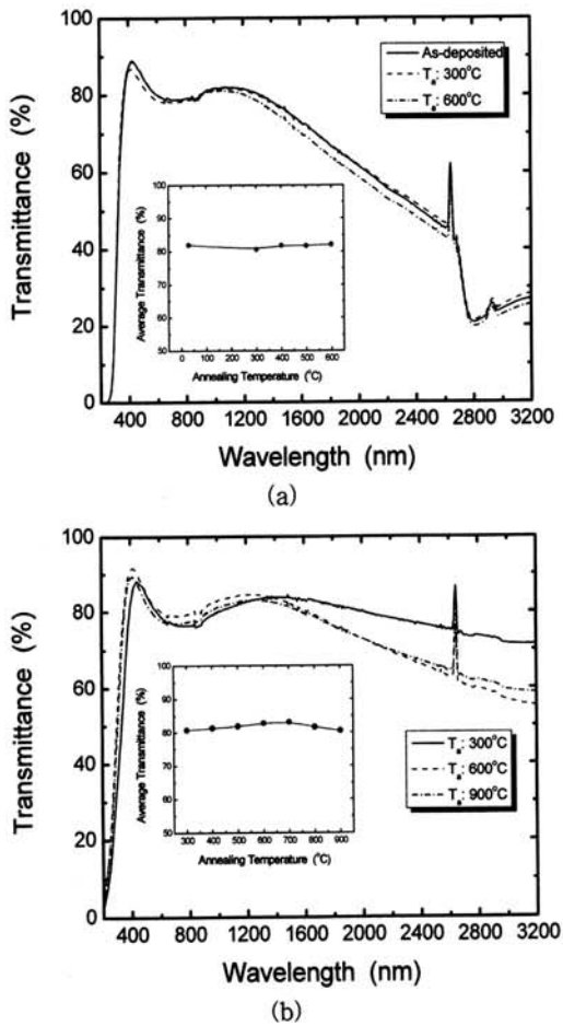
그림 8. 열처리 온도에 따른 SnO 2 :Sb 박막의 광 투과율: (a) 유리 기판; (b) 석영 기판. Fig. 8. Optical transmittance of SnO 2 :Sb films annealed at different temperatures: (a) glass substrate; (b) quartz substrate.
