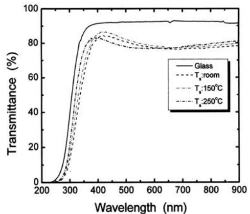
그림 5. 기판 온도에 따른 SnO 2 :Sb 박막의 광투과율. Fig. 5. Optical transmittance of SnO 2 :Sb films deposited at different substrate temperatures.
