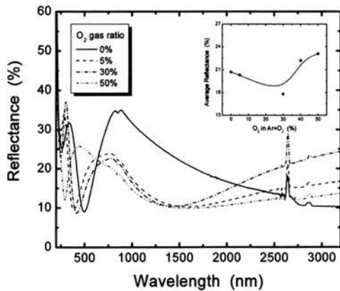
그림 3. 산소 가스 비에 따른 SnO 2 :Sb 박막의 반사율.
