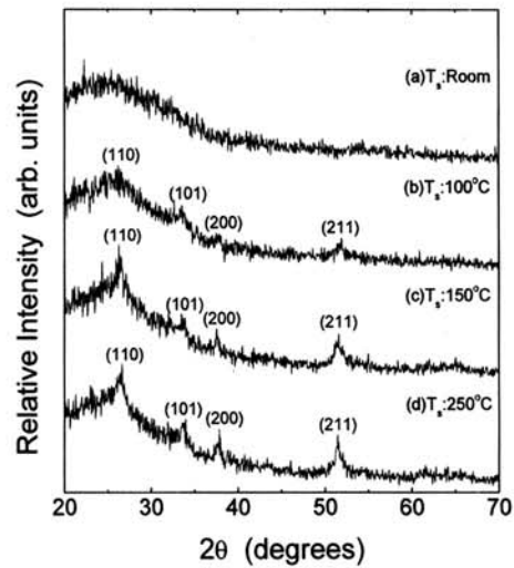
그림 4. SnO 2 :Sb 막의 기판온도에 따른 XRD 패턴. Fig. 4. X-ray diffraction pattern. XRD patterns of SnO 2 :Sb films deposited at various substrate temperatures.
