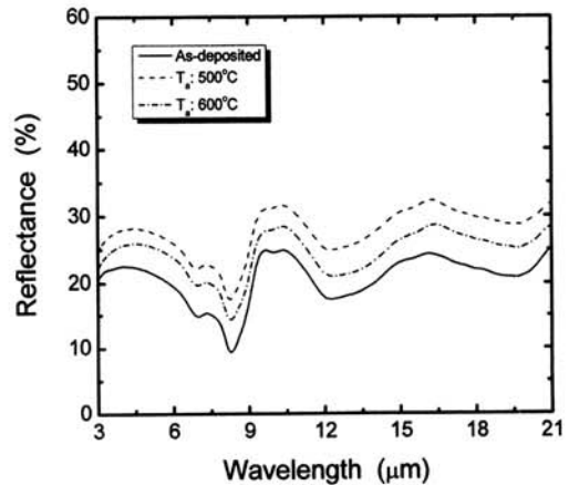
그림 9. 열처리 온도에 따른 SnO 2 :Sb 박막의 적외선 영역에서의 반사율. Fig. 9. IR reflectance of SnO 2 :Sb films deposited on glass substrate as a function of annealing temperature.
